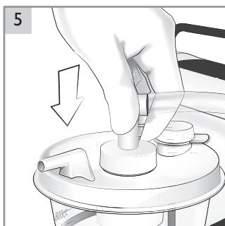
5 Slut den HVIDE kobling til koblingen på vakuumporten på beholderen.
